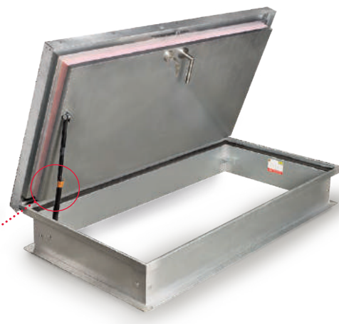
plynový píst s pojistkou proti svěvolnému uzavření víka
